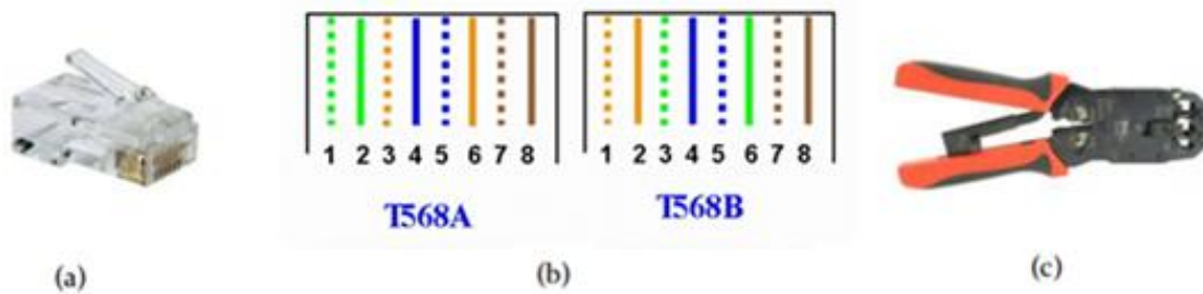
Figure 2. (a) Connecteur RJ45 (b) Schéma T568A et T568B (c) une pince pour connecteur RJ45.
