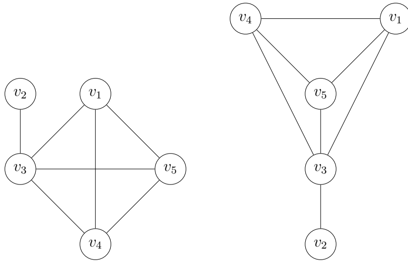
FIGURE 1.2 – (a) Une représentation non plane du graphe G et (b) sa représentation plane
