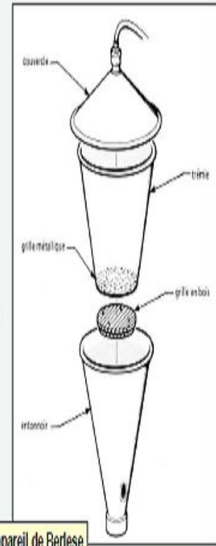
Appareil de Berlese
