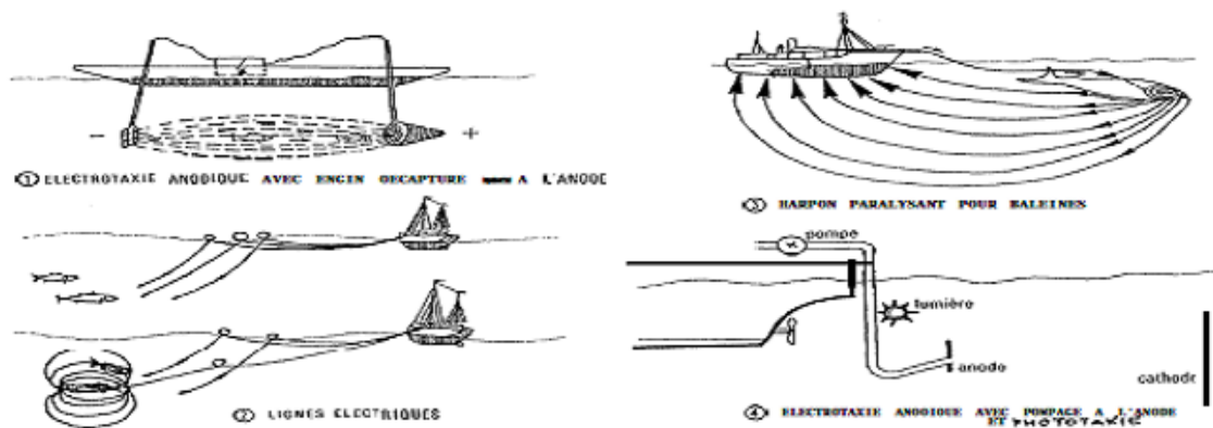
Figure 11.- engins électrifiés
