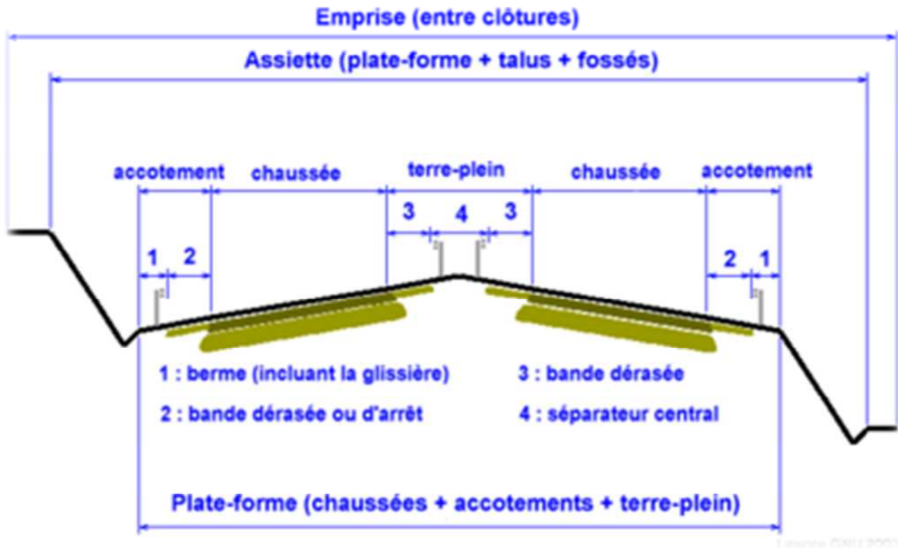
Schéma d'une coupe d'autoroute source Google images
