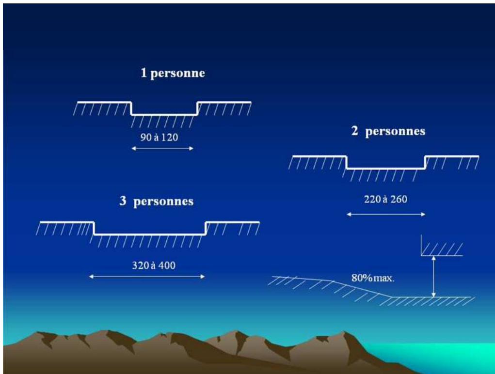
Dimensions accès piétons source : Exposé sur VRD/ EPAU / Kerrouche .M et Toumi. A
