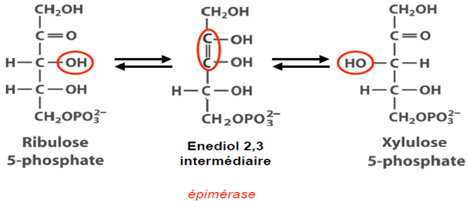
figure 5: réaction d'épimérisation
