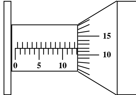
Lecture : 13,12 mm
