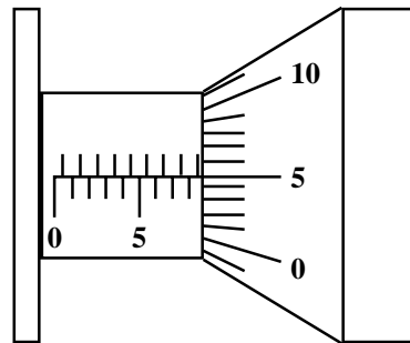
Lecture : 8,55 mm
