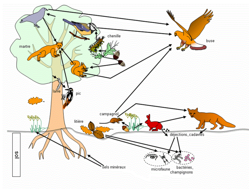
réseau trophique
