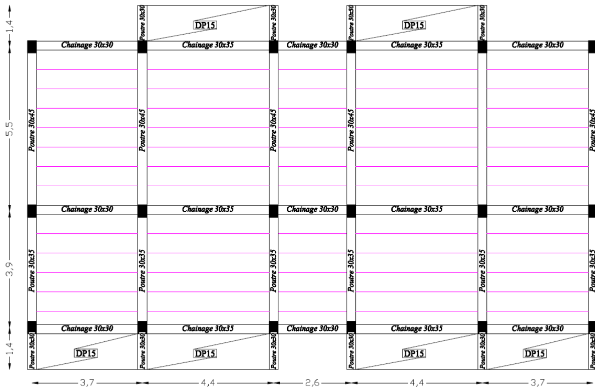
Plancher terrasse : Niveau = 18.87 m
