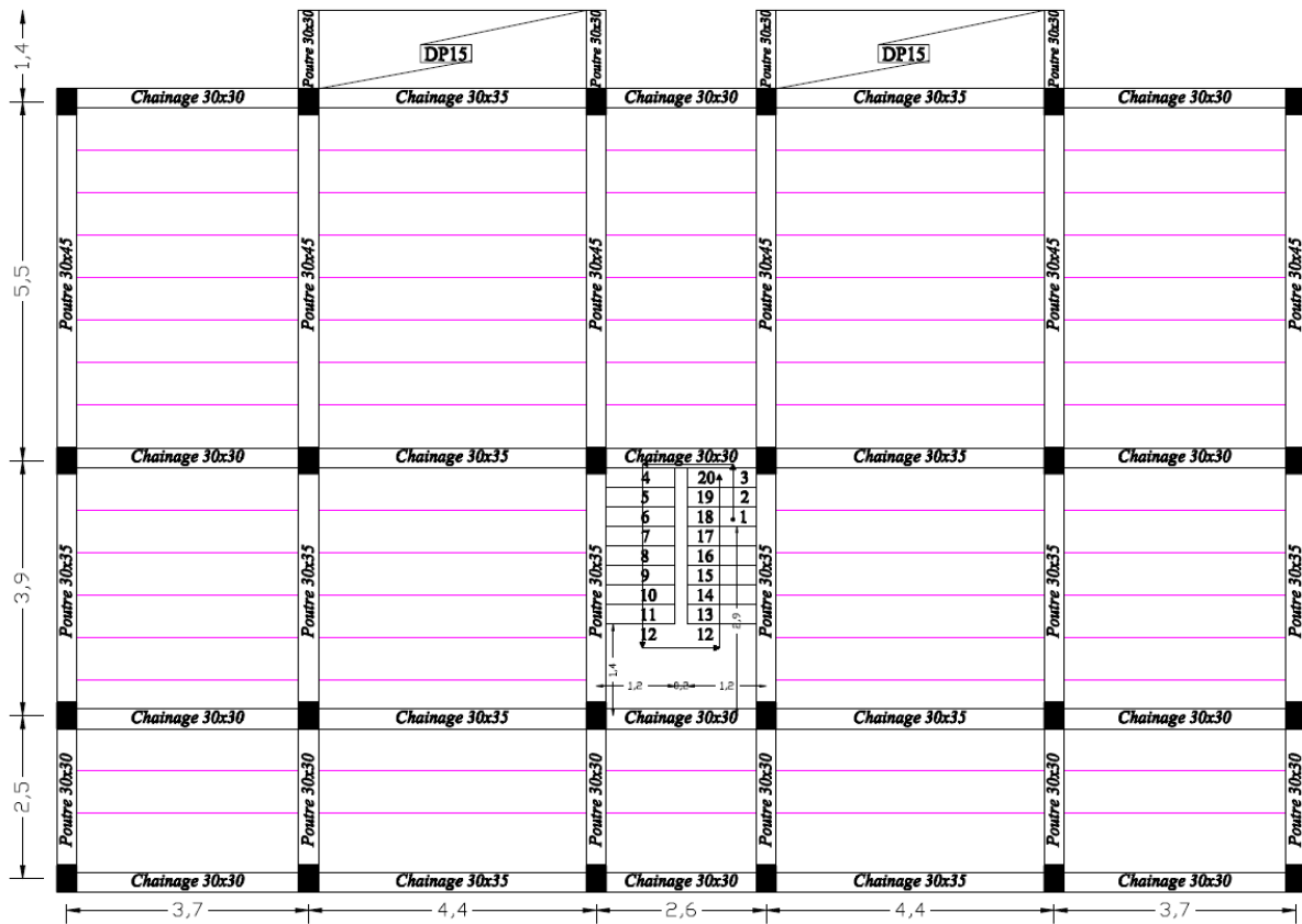
Plancher RDC : Niveau = 3.57 m
