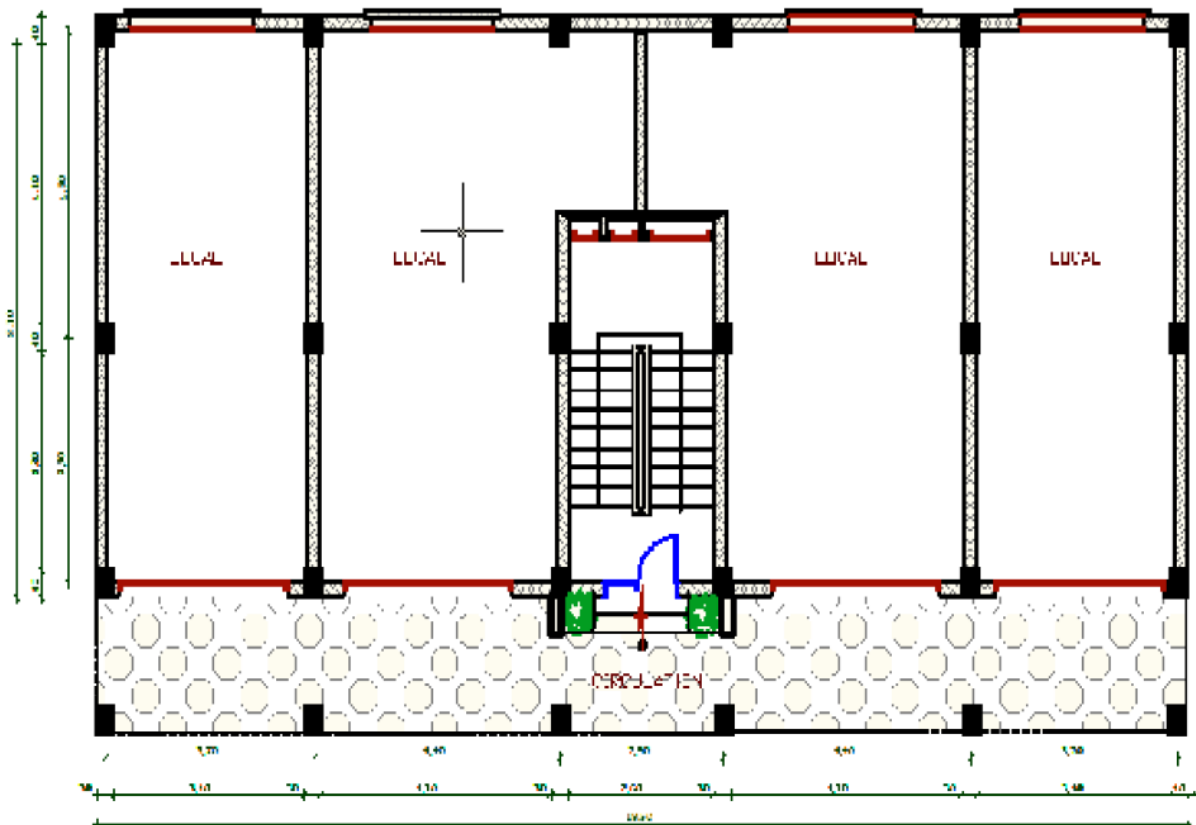
Fig. I.1: Vue en plan du réz de chaussée
