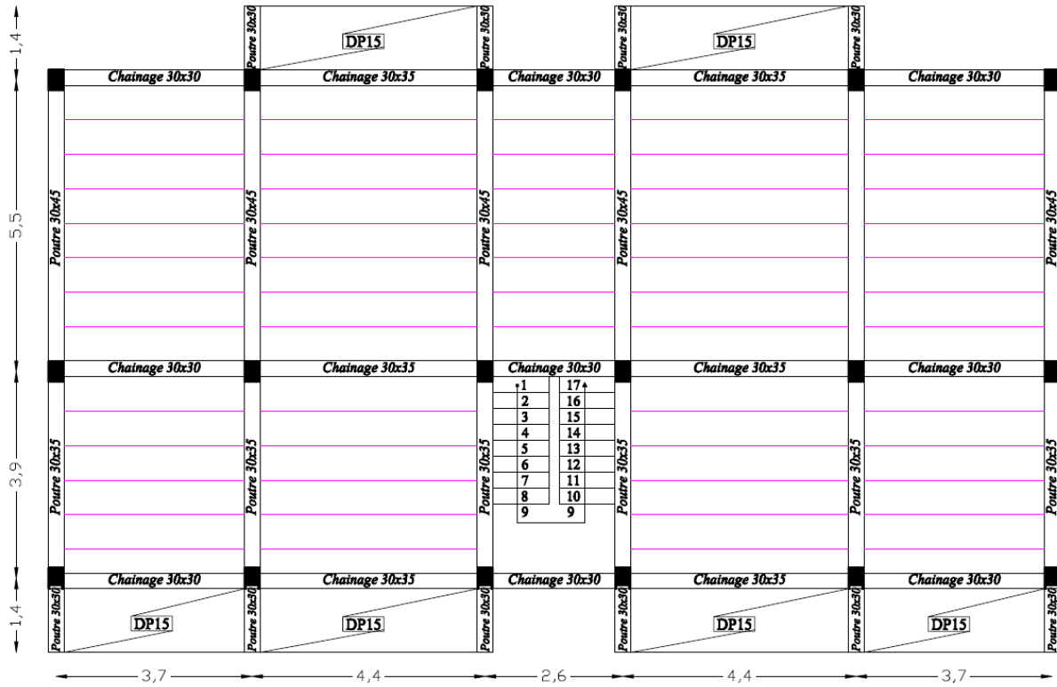
Plancher étage courant : Niveau = 6.63m + 9.69m + 12.75m + 15.81m
