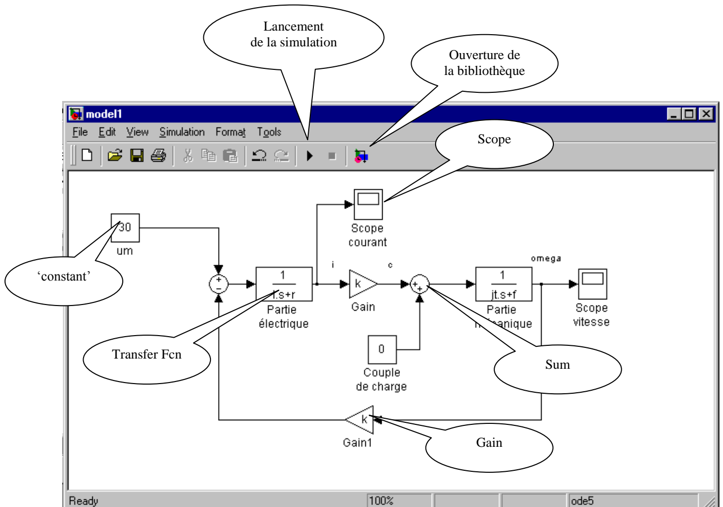
Figure 2 : Modèle de simulation associé au moteur à courant continu
